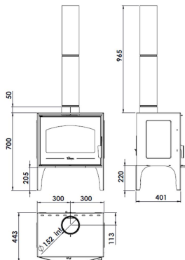
Abbildung 1 Abmessungen des Geräts in mm CALPE
