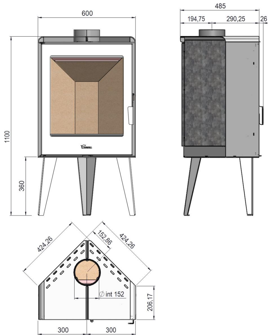
Abbildung 2 Abmessungen des Geräts in mm Atlantic 610R
