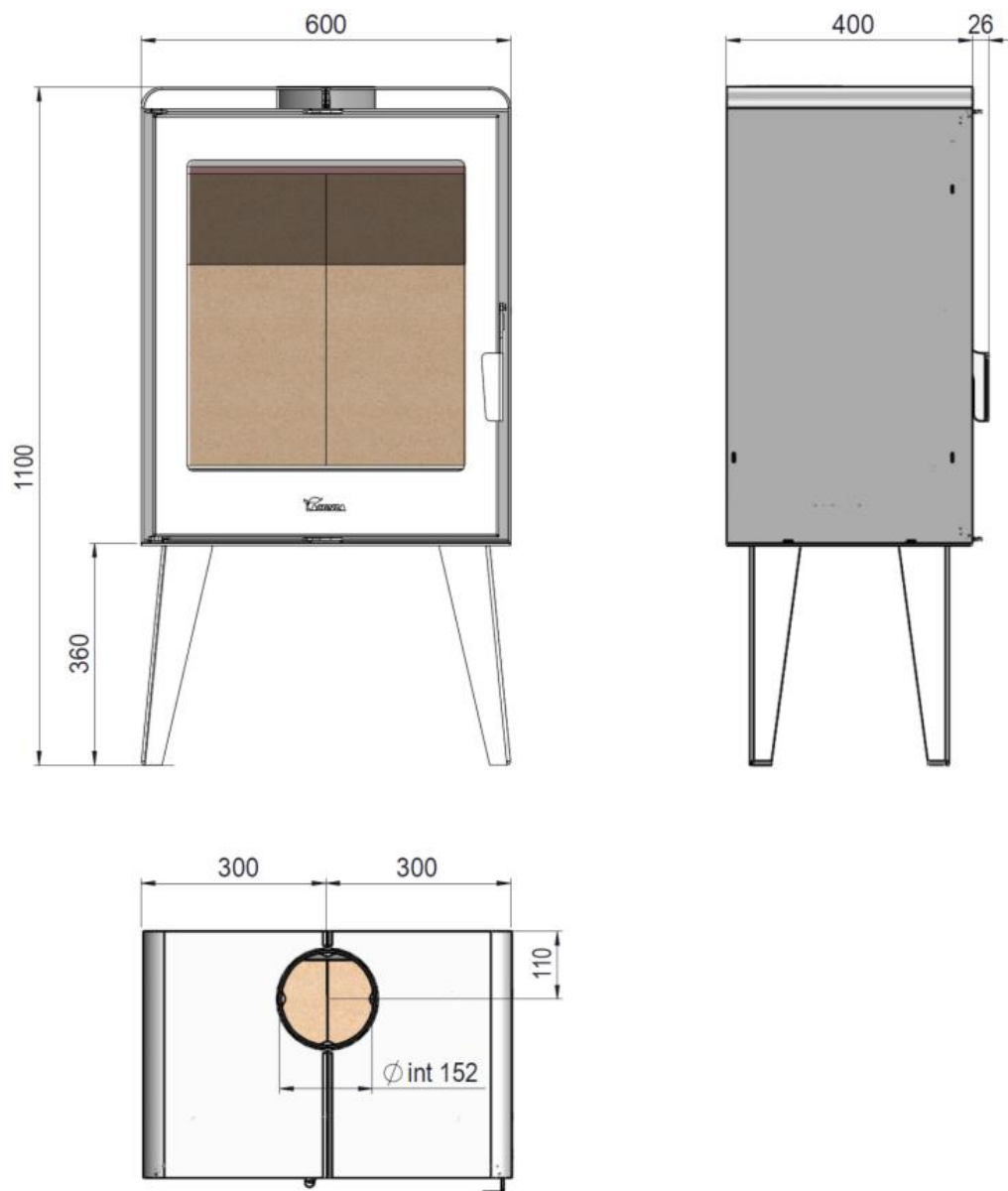
Abbildung 1 Abmessungen des Geräts in mm Atlantic 610
